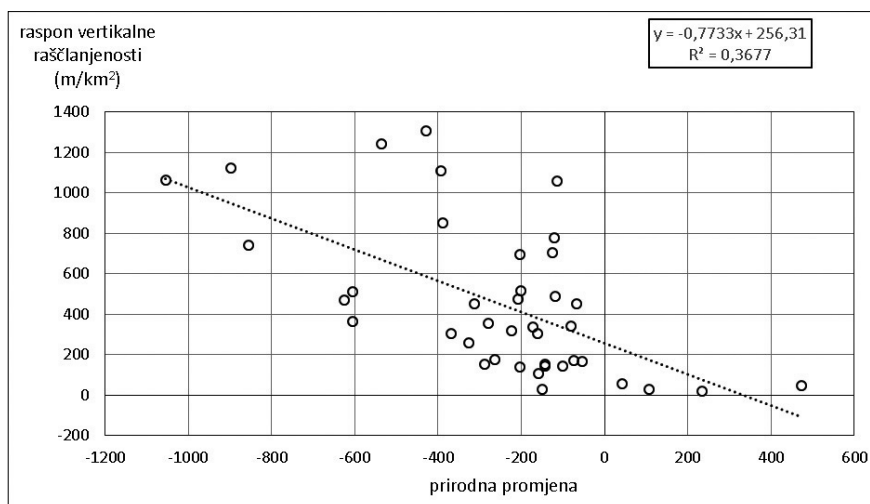
Sl. 9 Povezanost raspona vertikalne raščlanjenosti i prirodne promjene u analiziranim općinama.
