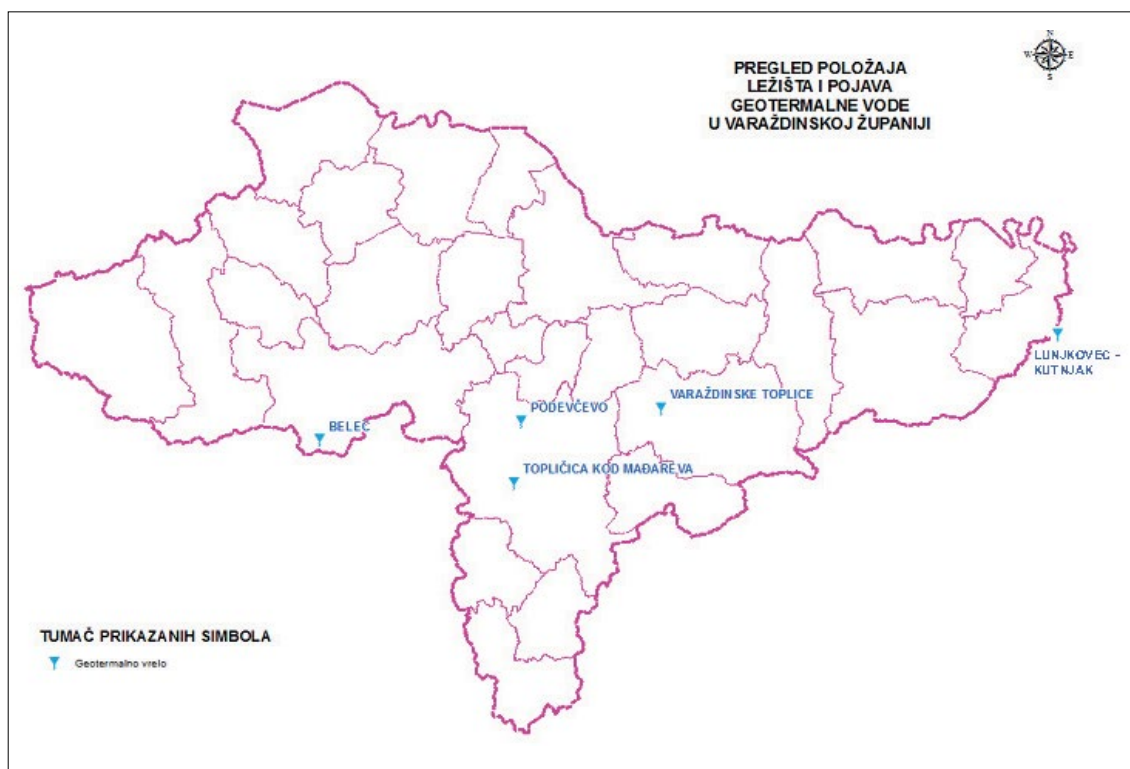
Slika 2. Pregledna karta ležišta i pojave geotermalne vode na području Varaždinske županije
