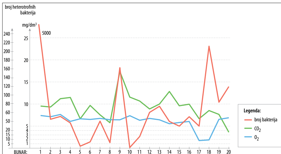
Grafikon 3. Odnos broja heterotrofne bakterije, otopljenog kisika i ugljik (IV) oksida u bunarskoj vodi Virja tijekom 1987. godine
