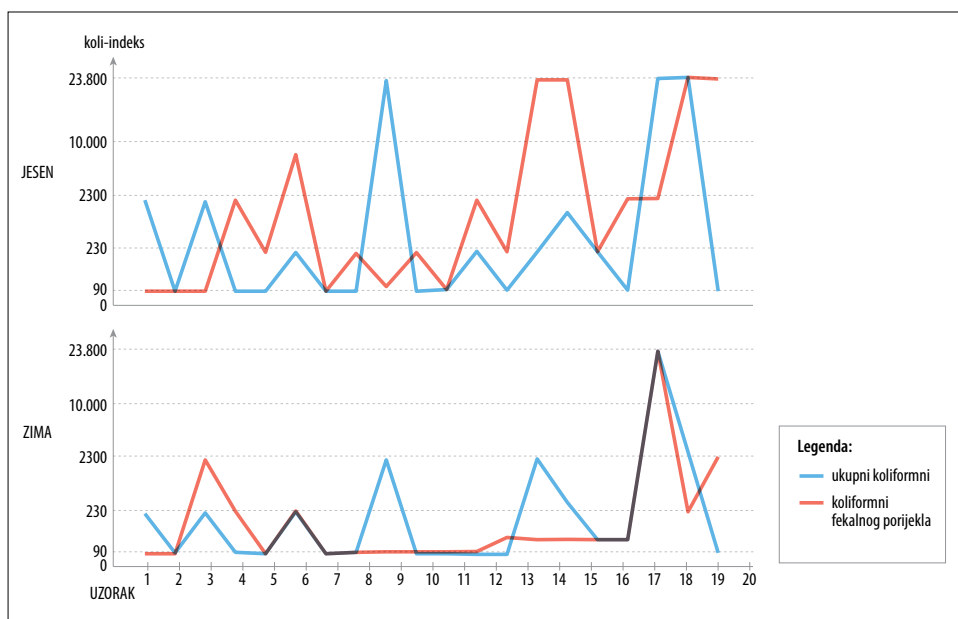
Grafikon 2. Odnos koli-indeksa ukupnih koliformnih bakterija i koliformnih bakterija fekalnog porijekla u bunarskoj vodi Virja u 1987. godini
