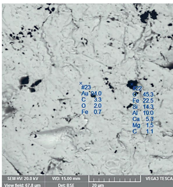
Slika 11. Elektronsko mikroskopska slika površine zrna zlata. Primjećuju se tamni uklopci željezovitog aluminosilikata, vjerojatno djelomično oksidiranog piroksena ili amfibola, čija je maksimalna veličina oko 2 mikrometra. Analizirana zrna zlata pokazuju vrlo visoku čistoću i preko 95% Au, koje je ovdje legirano s vrlo malim postotkom željeza
