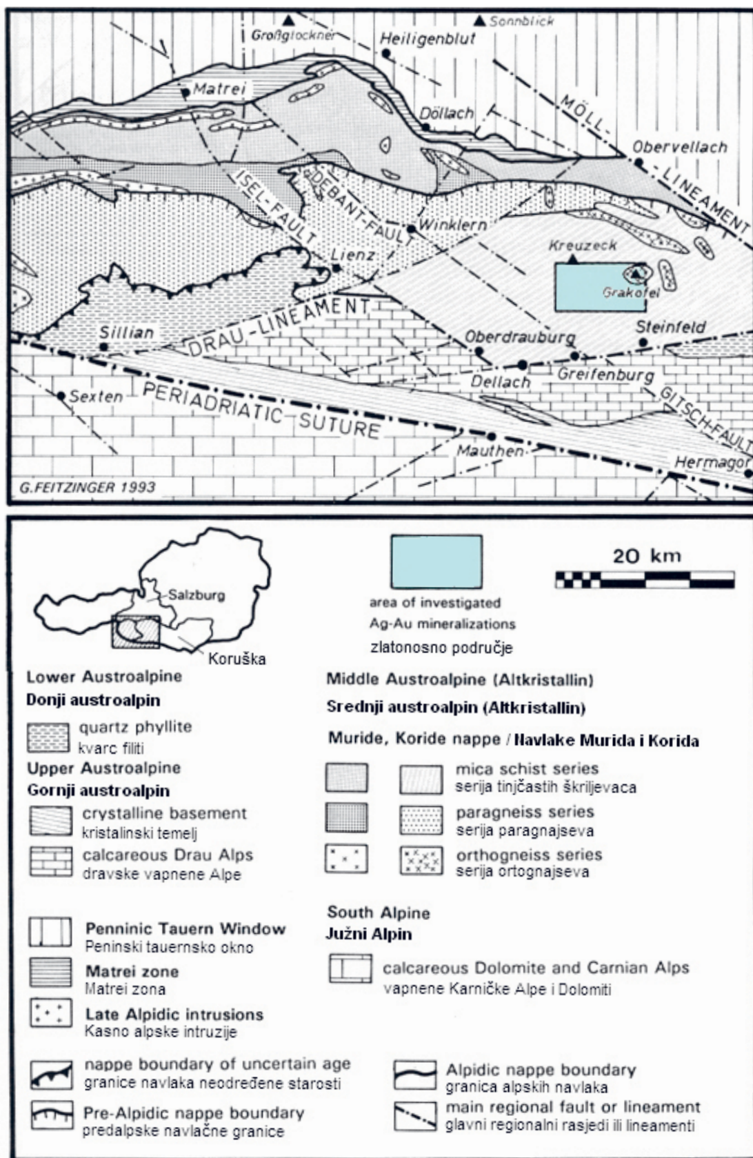
Slika 6. Geološka skica Kreuzeg planina, kao dijela južnog dijela Austroalpina unutar Peninskog Tauern okna (prema TOLLMANNU, 1977.)
