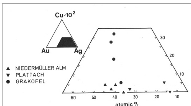
Slika 9. Sastav Au-Ag-Cu legura u Plattach, Niedermülleralm i Grakofel rudnom području prikazan u ternarnom dijagramu (preuzeto iz FEITZINGER i dr., 1995.)
