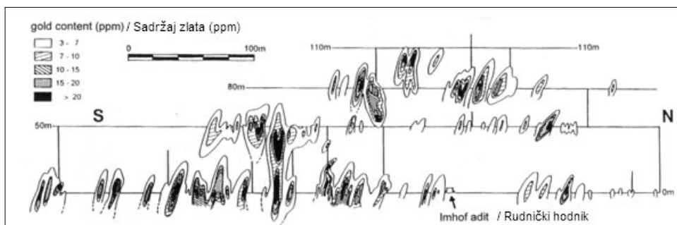
Slika 8. Zonalna distribucija zlata uzduž rudnog profila s orudnjenim žilama (Kuperwieser žila, u području Siglitz)
